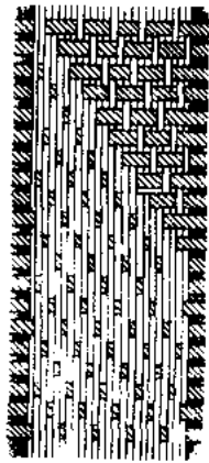
缎组织示意图
