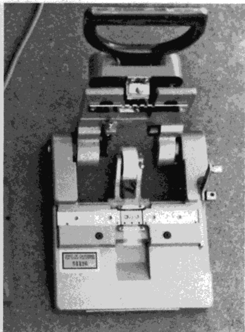
图 1-12 一种影片裁切机,可以用来切断底片并连接起来。其中有刀片可以切断底片,并有凹槽可以将两段底片固定住,再接合后即可完成一个剪接动作。这部裁切机会按照底片上的片孔,在接合用的特殊胶带上,打出和片孔一模一样的洞。
