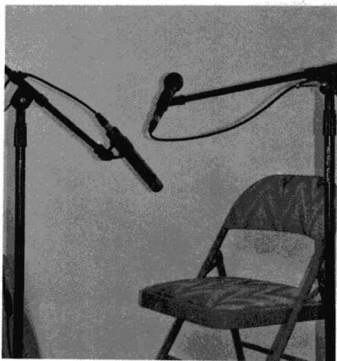
图 8-9 这个麦克风架设可用在歌手兼吉他手的表演者身上。一支麦克风在嘴巴旁边,一支则在吉他的音箱前方。
