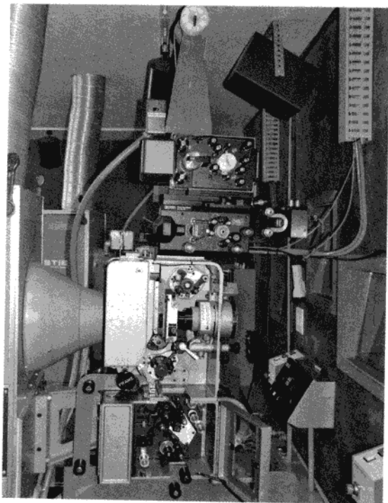
图 14-6 这个放映机的声音系统中，容纳有五种不同类别的声音。最上面是 SONY 的 SDDS 系统，中间是 DTS，会连接到外接的 CD-ROM。邻近这区域的是数字杜比系统。在下方有光学声音的读取设备，另外还有磁头，可以读取比较旧式的磁性声带胶片。
