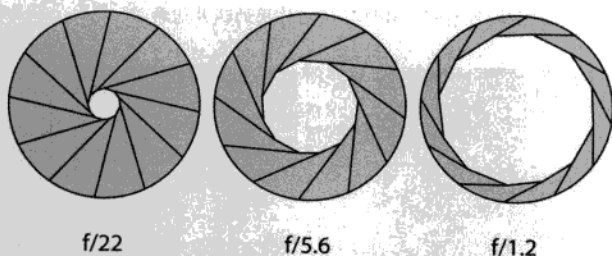
图3-20 镜头光圈中的金属薄片,可以打开或关闭不同光圈系数的光圈。开口愈小,光圈档位的数字愈大,进到摄像机的光线也就愈少。镜头的灵敏度是由最大光圈时进入的光线量来决定的。也就是说,一个最大光圈f/1.2的镜头,就比最大光圈f/2的镜头要更灵敏。
