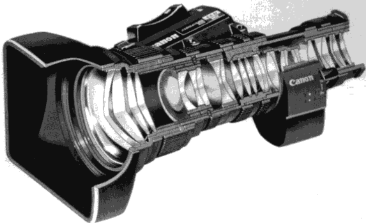
图 3-18 变焦镜头的解剖面,可看到内部许多不同作用的镜片组群。
