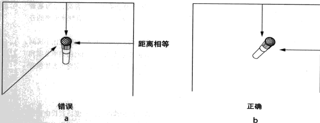
图 7-4 (a)这种麦克风放置方式,因为和墙壁平行,且间隔距离相同,很容易造成相位问题。(b)放置位置较佳,因为麦克风和各墙面是有角度的,离墙壁较近。
