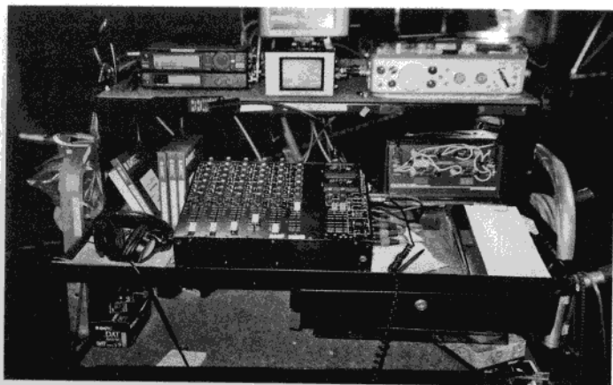
图 8-10 这个混音器包括左上方的 DAT, 右上方的纳格拉, 以及便携式混音操作台。它可以使用在多种电影和电视制作上, 同时还可把声音传送到摄录放一体机上。
