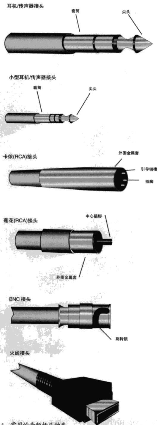
图 7-14 常用的音频插头种类
