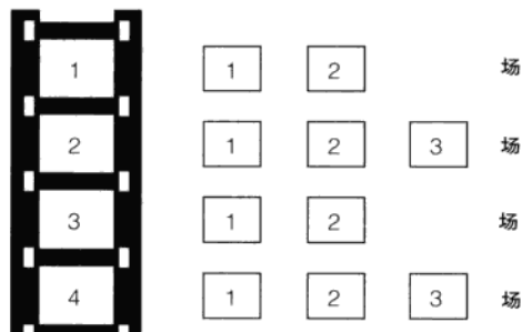
图 10-5 三二抓片法可以补偿胶片(每秒 24 格)和电子影像(每秒 30 个图框),在速度上的差异。胶片的每格画面会轮流地先扫描成 2 个场(一个图框),之后是 3 个图场(一又二分之一一个图框),因此胶片 24 格就相当于电子影像 30 个画框。
