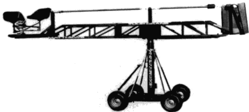
图 3-25 升降设备,要注意是否有装置摄影(像)机和操作者所坐的空间。
