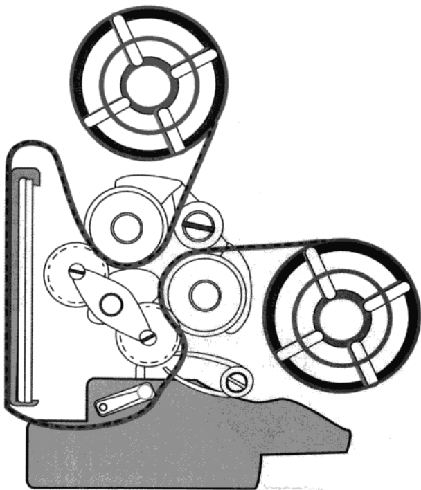
图 3-12 胶片在摄影像机中的安装上带方式。
