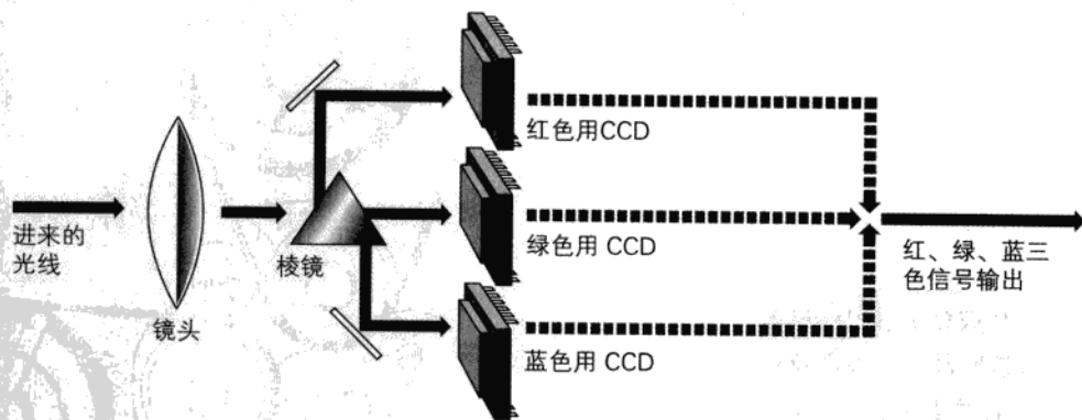
图 3-13 光线经过镜头进来后,被棱镜分解成红、绿、蓝三原色。分解后的信号,就被传送到适合的红、绿、蓝三个 CCD 中。最后,会有编码器把这些区别开的色彩信号再结合,产生全色彩的影像。
