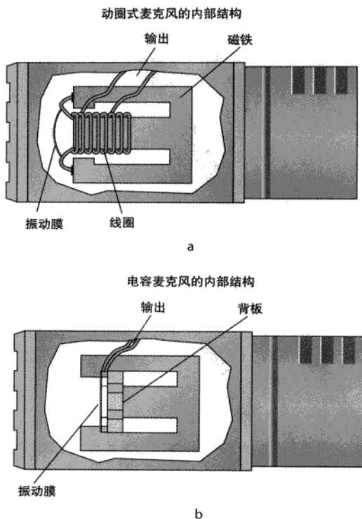
图 7-9 两种常用麦克风类型的构造:(a) 动圈式麦克风;(b) 电容器式麦克风。
