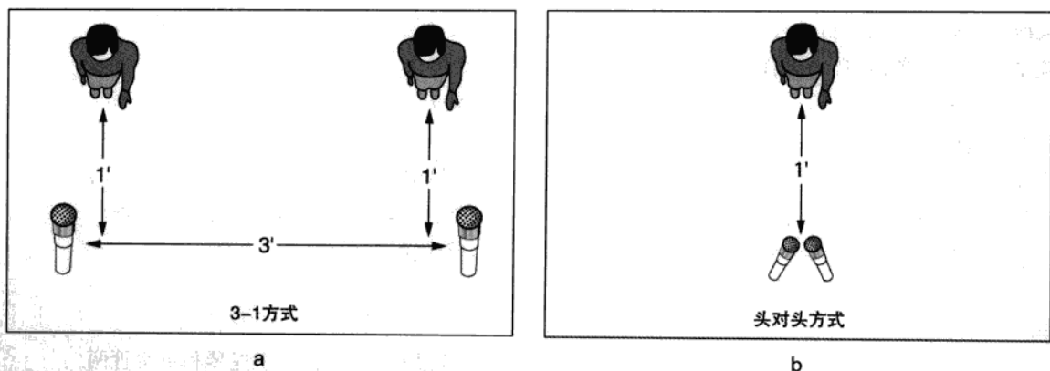
图 7-3 有两种主要方法来避免多支麦克风间的互相干扰。(a)3-1 方式呈现出如何以三倍距离原则放置麦克风;(b)头对头方式,则告诉你如何以面对面、头对头的方式放置麦克风。
