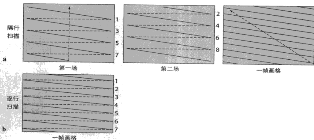
图 3-7 显示的是隔行扫描和逐行扫描的差别。(a)在隔行扫描时,单数的扫描线先行扫描,由左到右进行扫描。到了右边缘时,扫描线先遮盖,然后快速地折返回左边,再开始扫描下一条。所有单数扫描线,就构成了半个画面,也就是一个场(field)。之后扫描线进入了场消隐期(vertical blanking),让扫描线回到最上方开始双数扫描线扫描,再构成画面的另外一半。每个场扫描时间为 1/60 秒,两个场结合成一帧画格,也就是 1/30 秒。(b)在逐行扫描时,扫描线是按顺序连接着扫描,来构成一个完整的画格。
