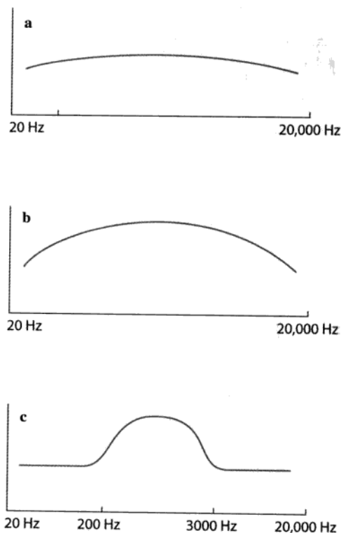
图7-2 这是麦克风或其他电子设备最普遍的三条频率曲线表。(a)图通常会认定是较平板的曲线,因为设备对所有频率都有相同的录制能力;(b)则代表设备对中间频率反应最佳,低频率和高频率次之;(c)则是在人类对话的频率上,有着最佳反应。
