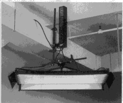
图 5-21 以高空夹安装固定妥当的高频荧光灯
