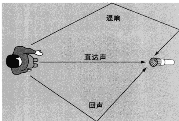
图 8-1 该图表现的分别是没有被任何表面反弹而直接被麦克风收到的直达声,经过一个表面反弹的回声,以及经过两个以上表面反弹的混响。
