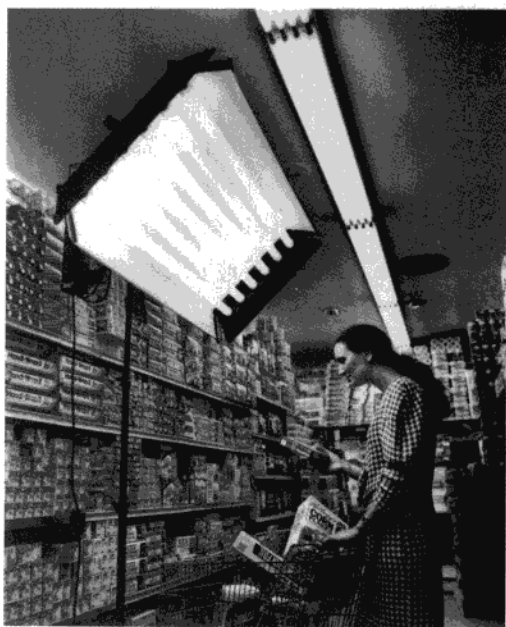
图 6-14 对本图中的女演员有可能和购物车一起移动的距离中,由高频荧光灯发出的柔和的光线是可以应付的。
