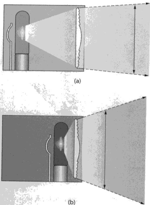
图 5-14 (a)灯泡这一点的位置离灯具前方镜片较远,所以产生聚光效果;(b)灯泡离灯具前方镜片较近,则是散光效果。
