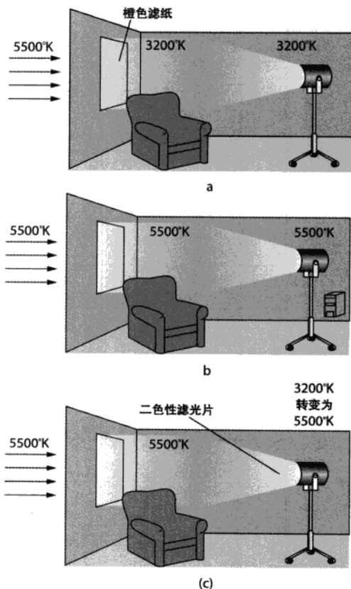
图 6-12 传统混合光源,有三种解决方式:(a)在窗户上张贴橘色 85 滤镜纸,这样可以把带有蓝色的日光修正至 3,200° K 的色温;(b)以日光平衡 5,500° K 的 HMI 灯具在室内使用,就可搭配由窗户进来的日光色温;(c)在灯光前装上蓝色的滤镜纸,也可以把 3,200° K 的色温,转变成 5,500° K,不过缺点是会大幅度地减少 3,200° K 灯具的光亮度。
