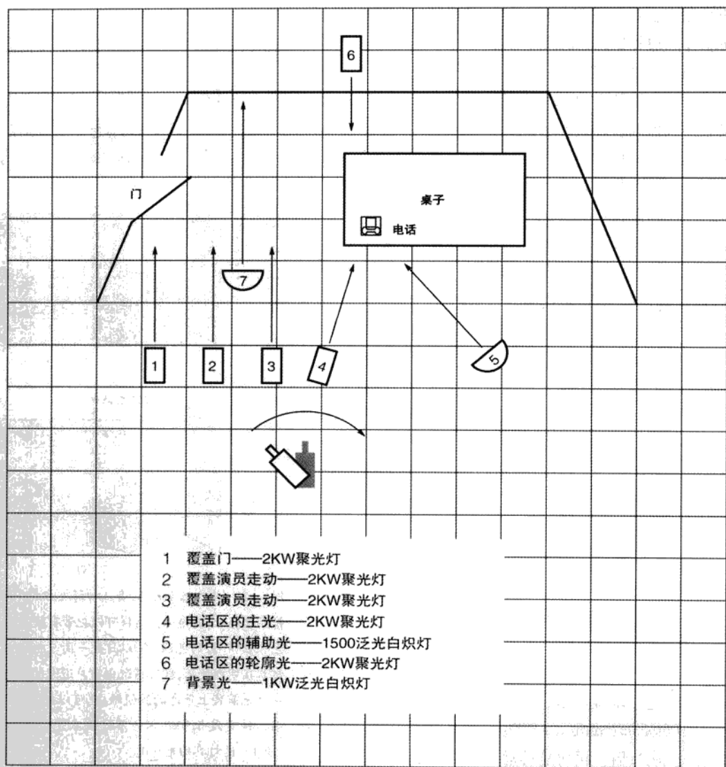
图 6-13 照明规划图,附注有灯光类型、亮度瓦数,以及每个灯具的作用。不过在这范例中,灯具是悬挂在铁架上。
