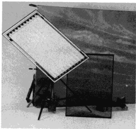
图 5-25 在高频荧光灯后方的光线漫射装置,当安装在灯具之上时,就可以有光线扩散效果。
