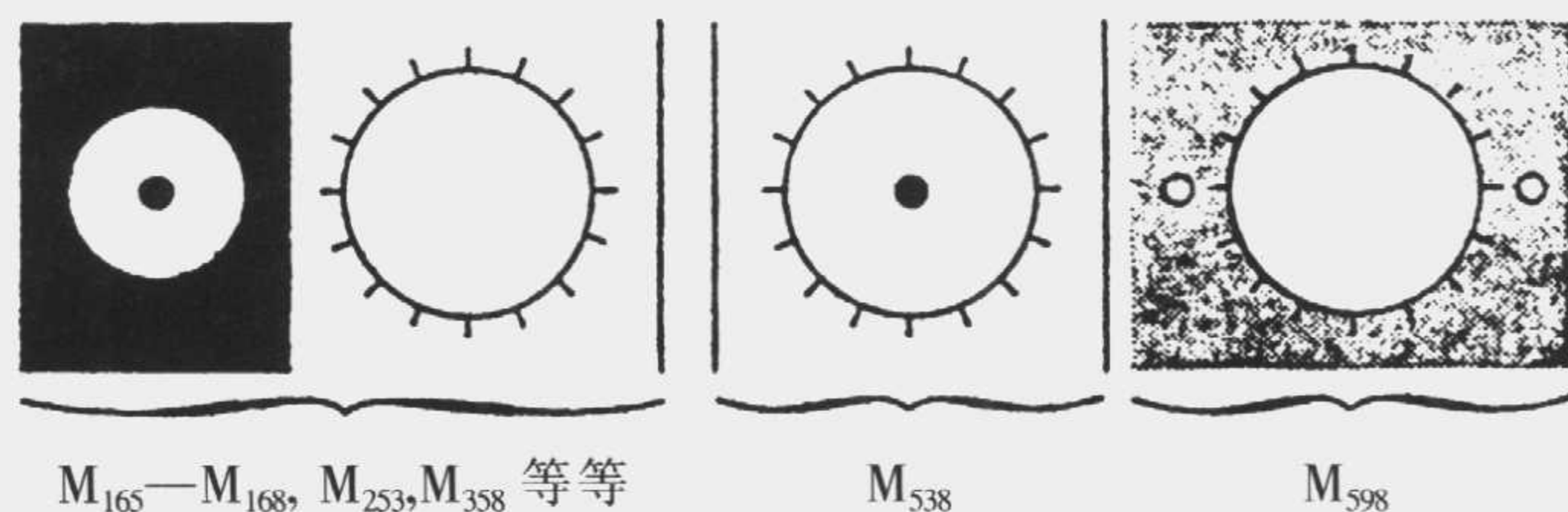
图 17 天体的转换
